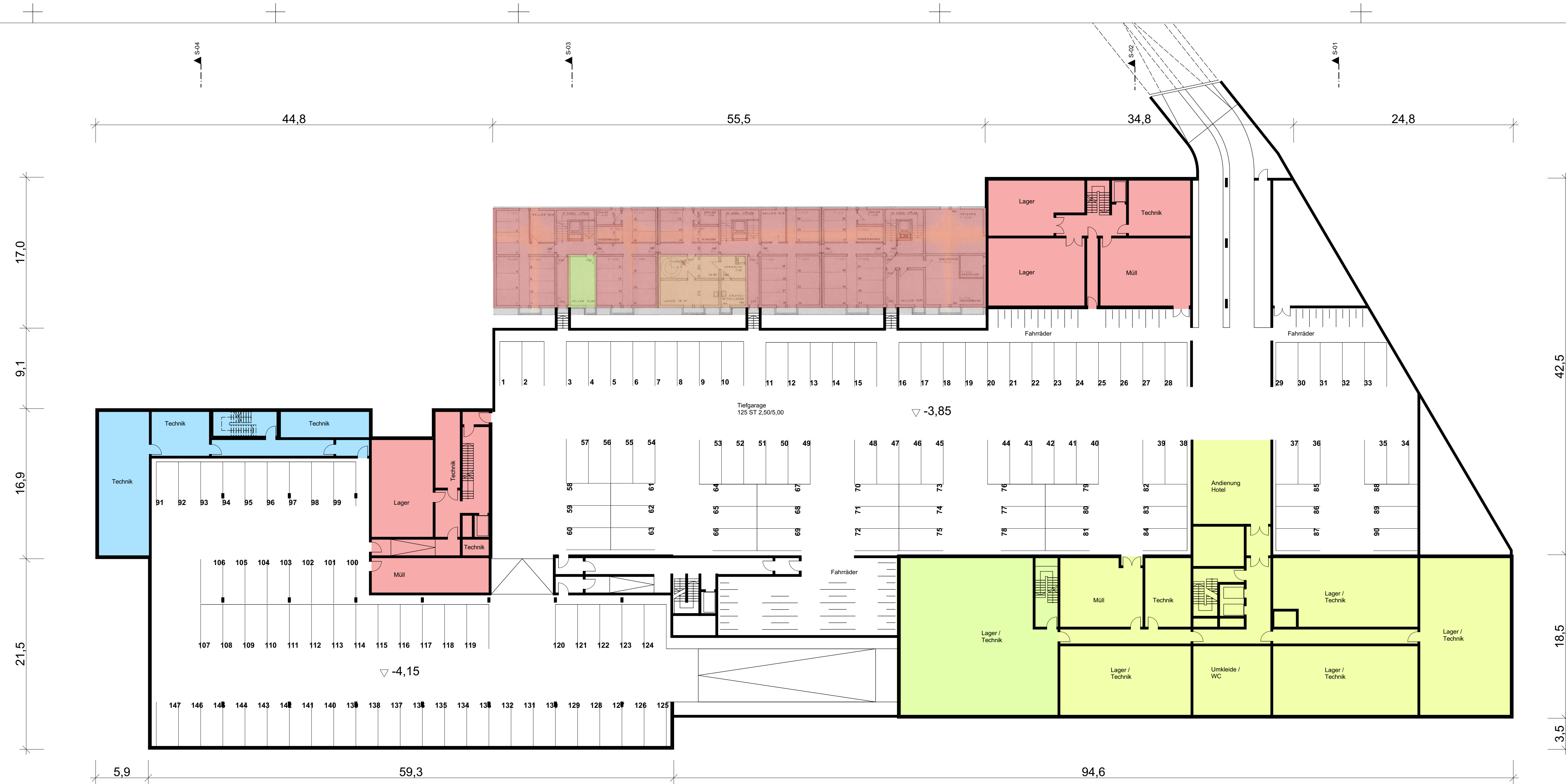
Grundriss 1. Untergeschoss M 1:250
